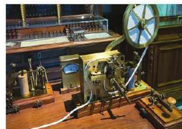
Hình 2.4. Máy điện báo
