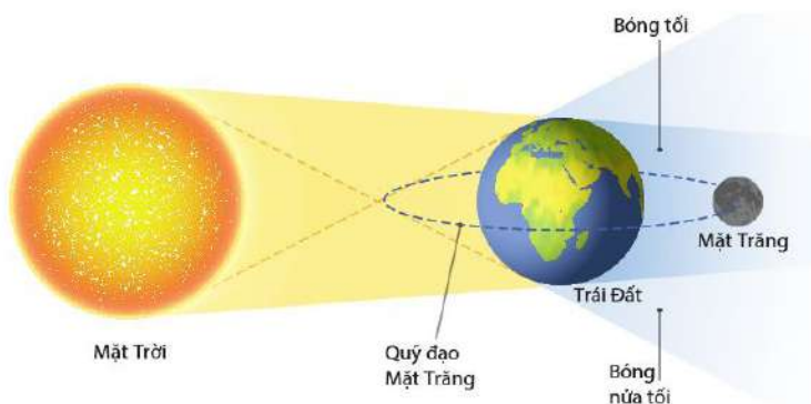
Hình 3.2. Sơ đồ giải thích nguyệt thực
